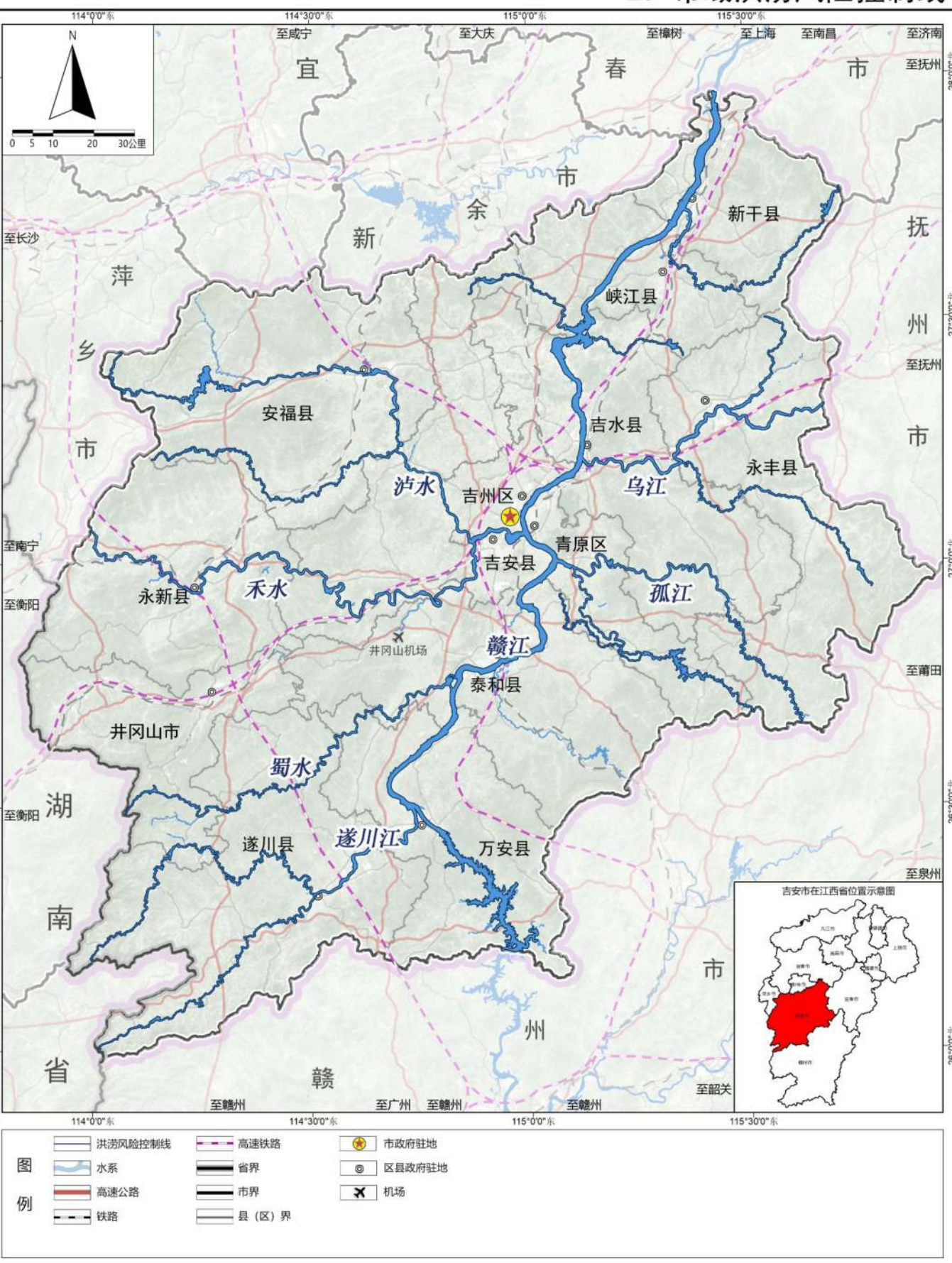
27-市域洪涝风险控制线
